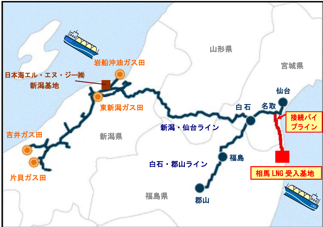
相馬 LNG 受入基地ならびに接続パイプライン 位置図
