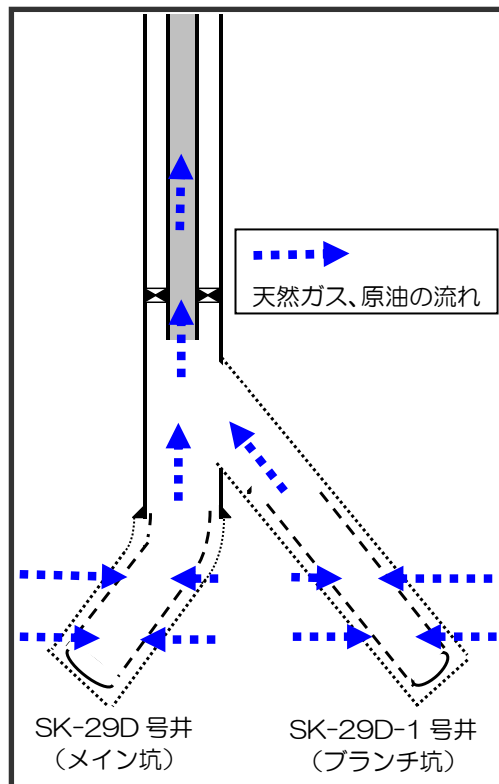
「マルチ・ブランチ坑井」イメージ図
